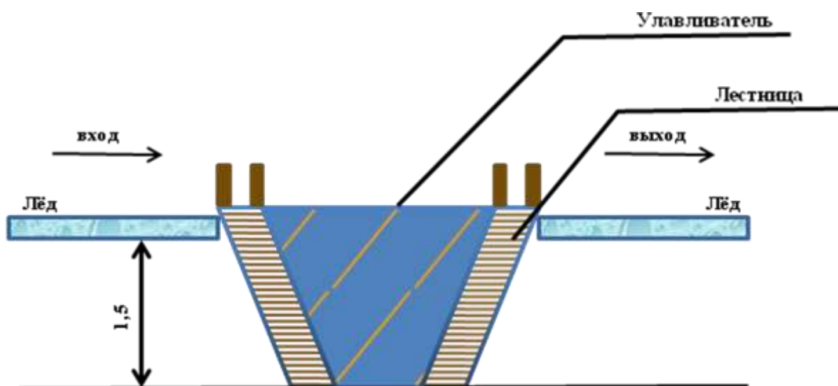
Схема оборудования купели (вход со льда)
